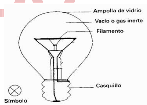
Lámpara incandescente
